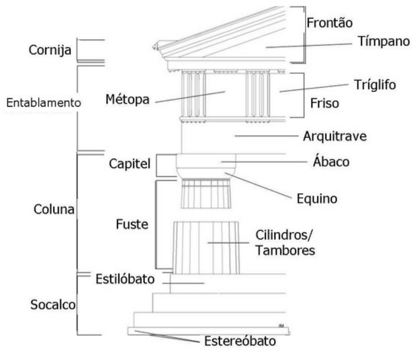
Estrutura da ordem dórica e jónica, respectivamente
