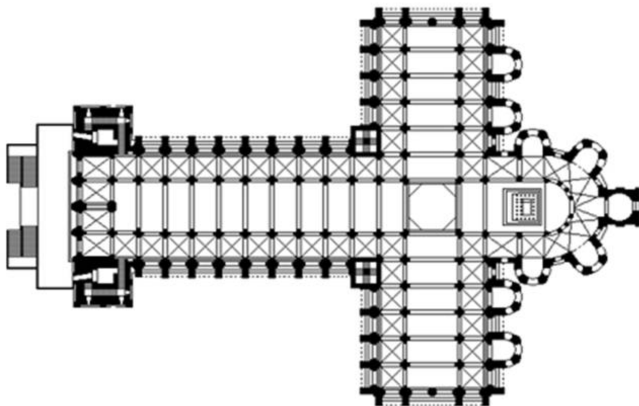
Planta de la Catedral de Santiago de Compostela (1075-1188)
